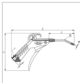
Pištolj vazdušni tip CB01-G(F)
