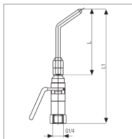
Pištolj vazdušni tip 321-90
