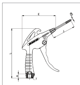
Pištolj vazdušni tip CA
